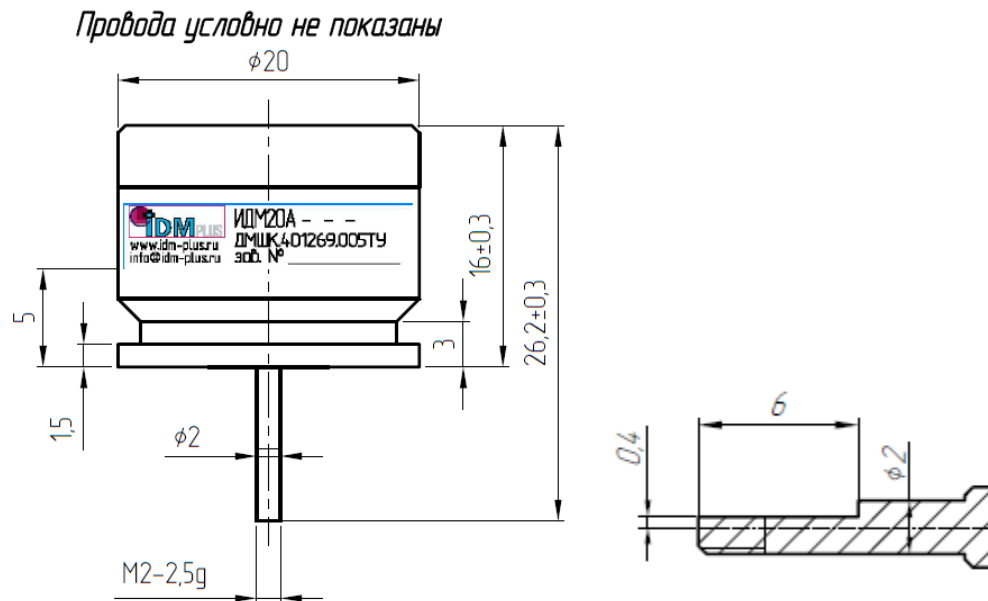
Рис. 4.2 – Исполнение с валом 2 мм
