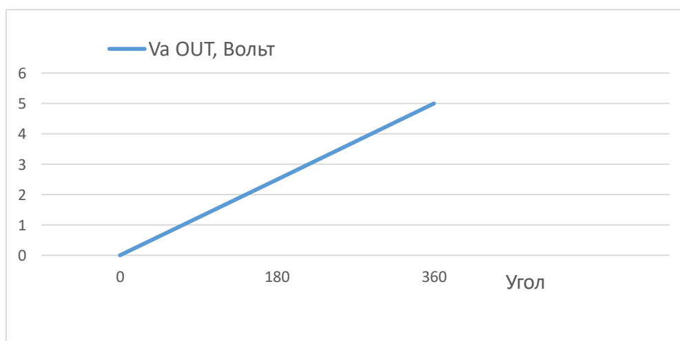
Рис. 8.1 – Аналоговый стандартный режим
