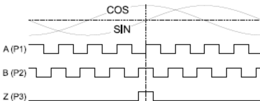
Рис. 7.1 – Инкрементальный
