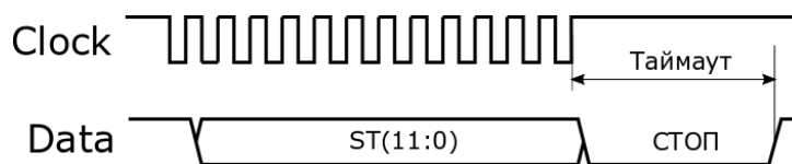
Рис. 6.2 SSI Протокол
