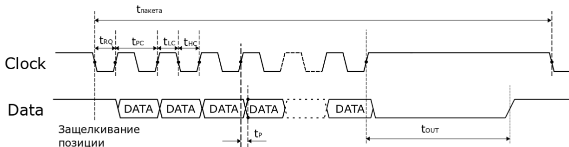
Рис. 6.1 Временная диаграмма SSI интерфейса
