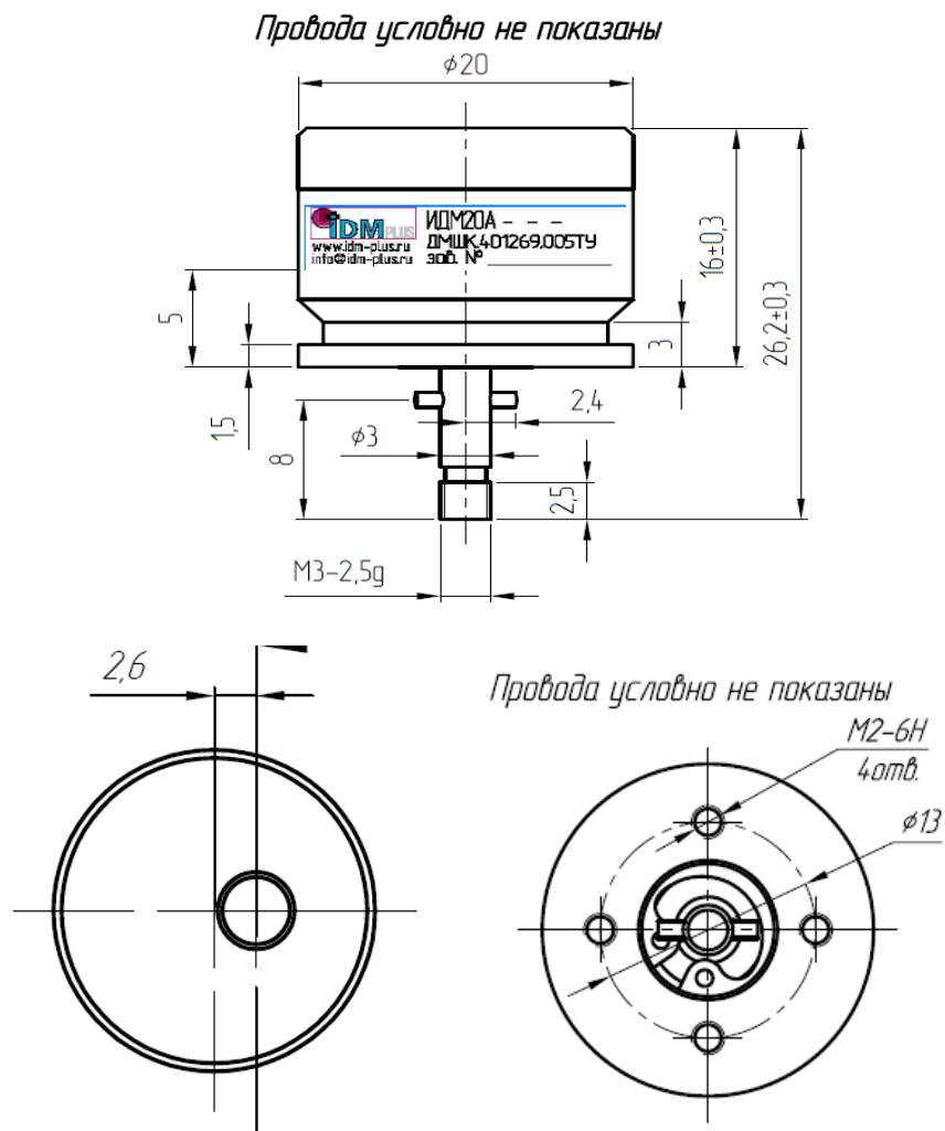
Рис. 4.1 – Исполнение с валом 3 мм
