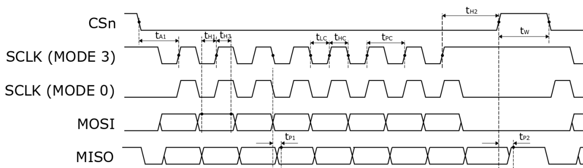
Рис. 5.1 - Временная диаграмма SPI интерфейса
