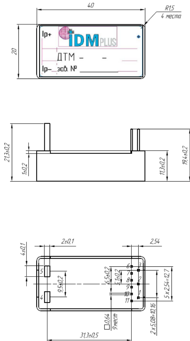
Рисунок 2.1 Габаритные, установочные и присоединительные размеры ДТМ для конструктивного исполнения 3.1
