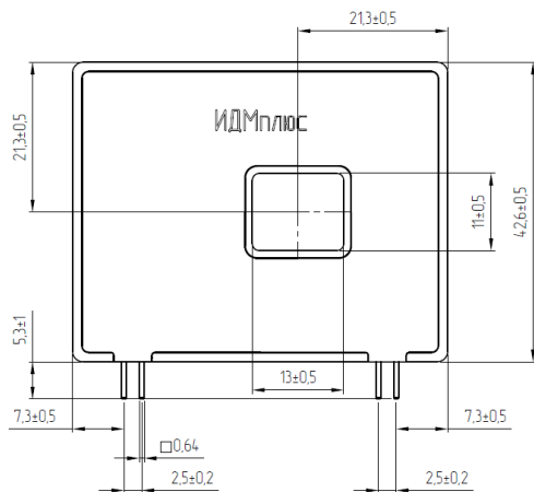
Рисунок 2 – ДТК-125, вид сбоку
